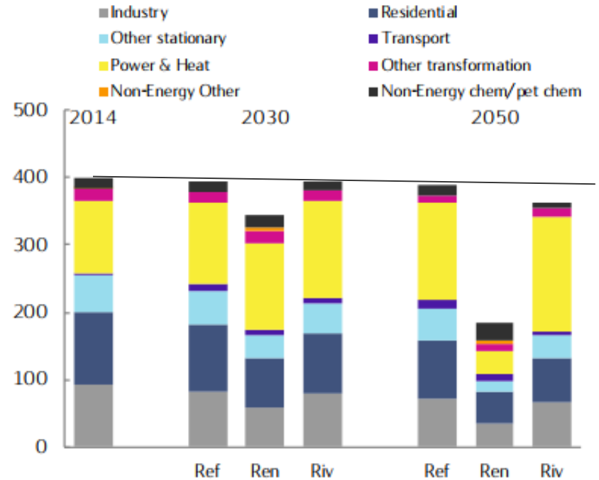
EU gas demand 2014-2050
